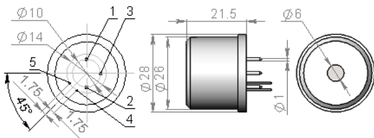
Рис.1 Размеры сенсора и схема расположения выводов 1 - индикаторный электрод 2 - вспомогательный электрод 3 - электрод сравнения 4,5 — выводы для нагрева(МГТФ)
